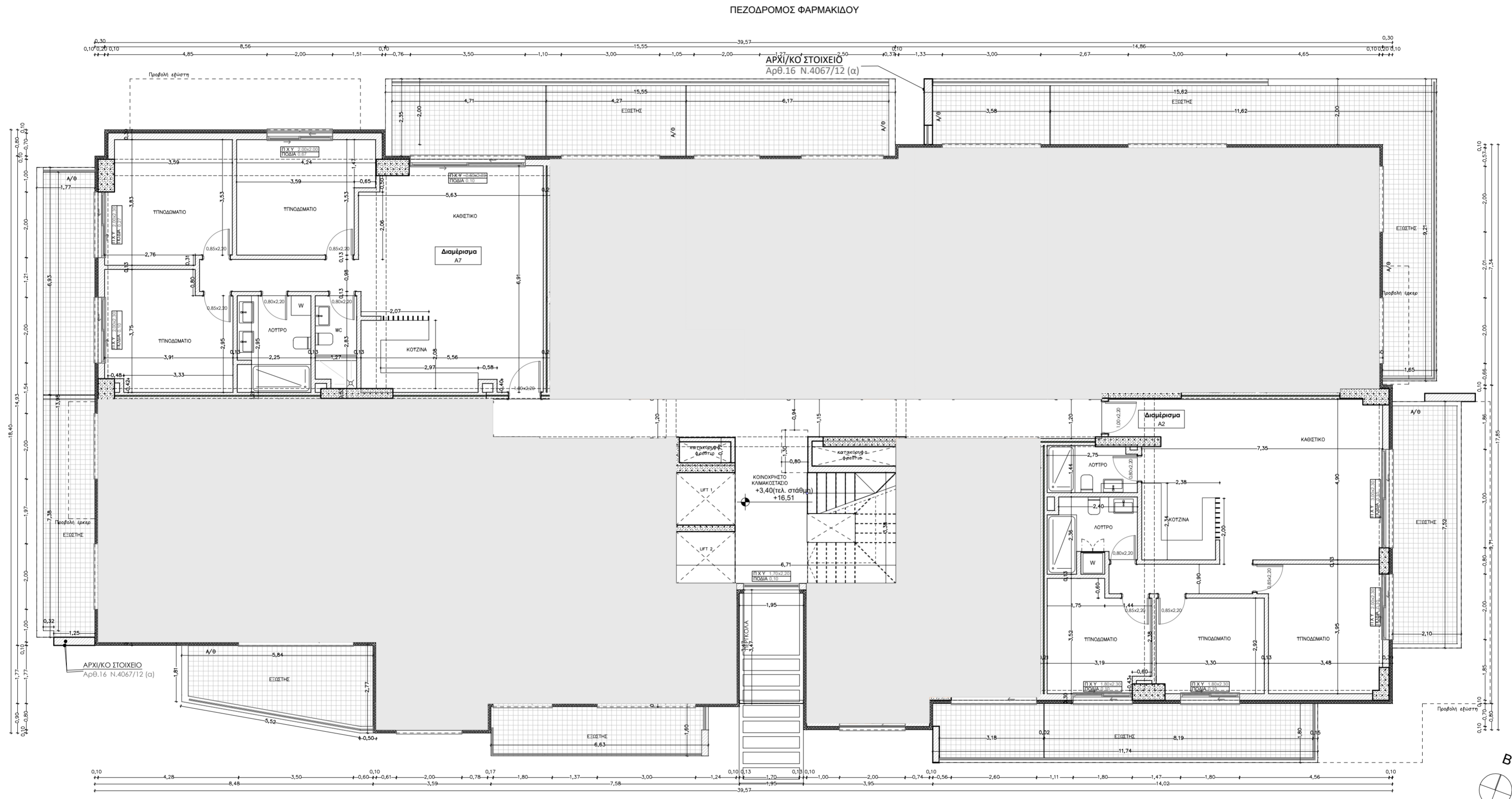
ΚΑΤΟΨΗ 1ου ΟΡΟΦΟΥ ΚΛΙΜΑΚΑ 1:100
