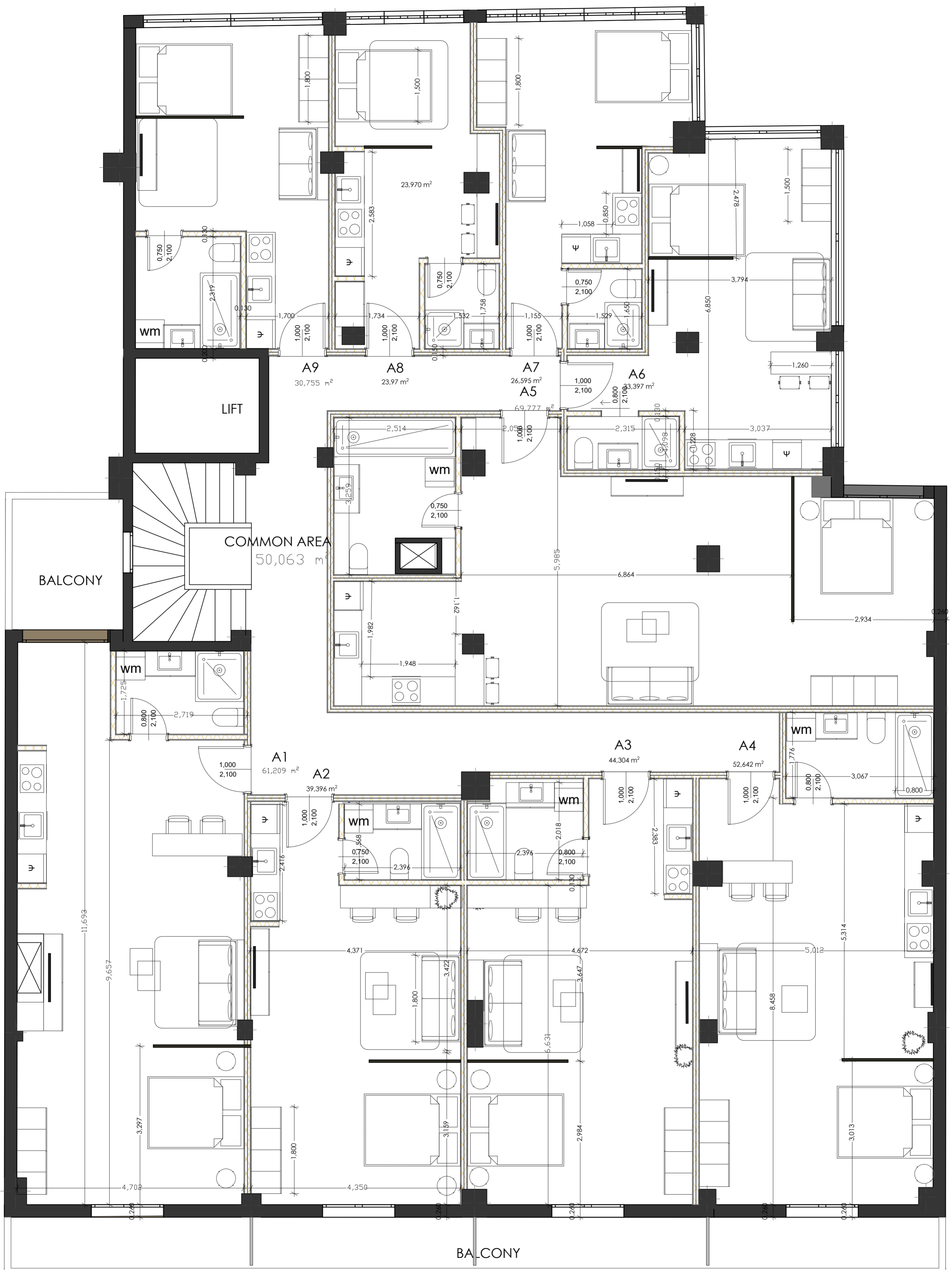
ΚΑΤΟΨΗ 1ου ΟΡΟΦΟΥ ΚΛΙΜΑΚΑ 1:50
