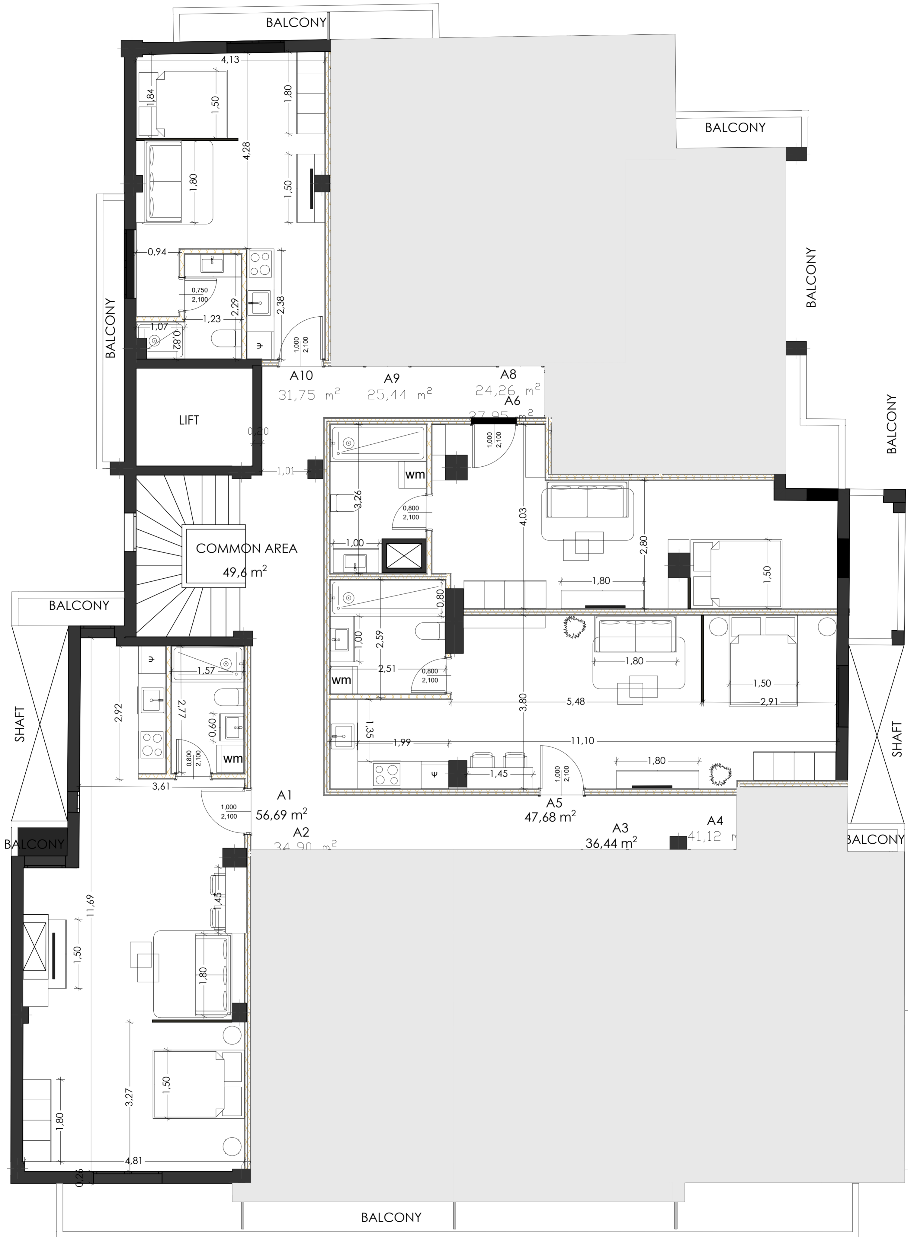
ΚΑΤΟΨΗ 2ου ΟΡΟΦΟΥ ΚΛΙΜΑΚΑ 1:50
