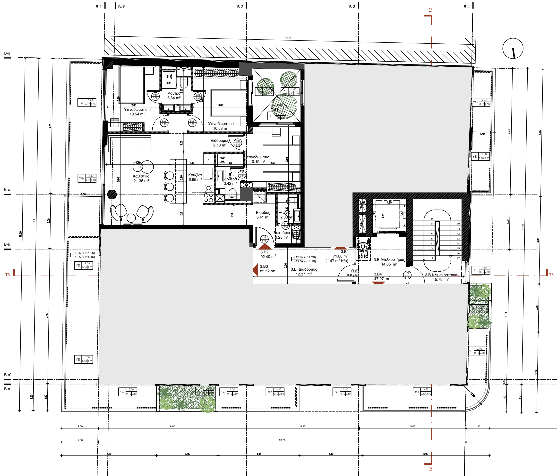
ΚΤΙΡΙΟ Β ΚΑΤΟΨΗ 4ου ΟΡΟΦΟΥ ΚΛΙΜΑΚΑ 1:100
