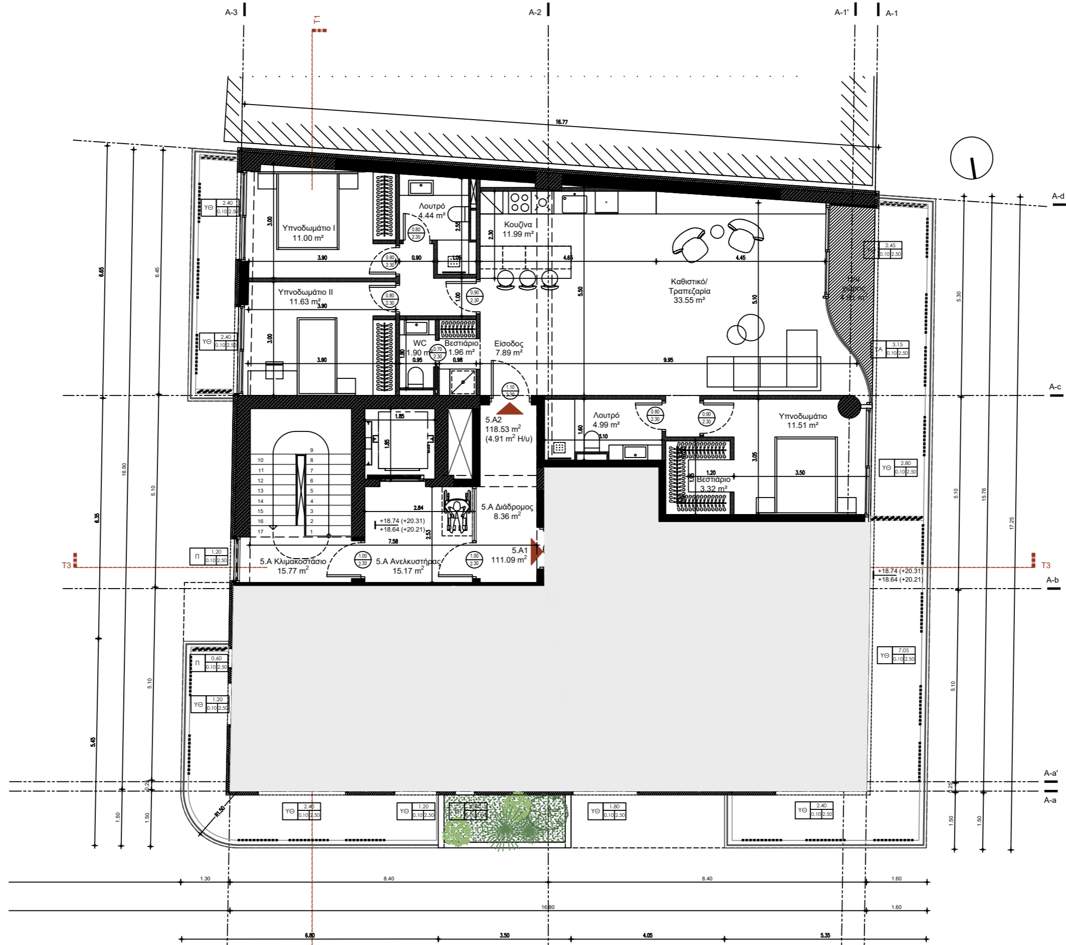
ΚΤΙΡΙΟ Α ΚΑΤΟΨΗ 6ου ΟΡΟΦΟΥ ΚΛΙΜΑΚΑ 1:100
