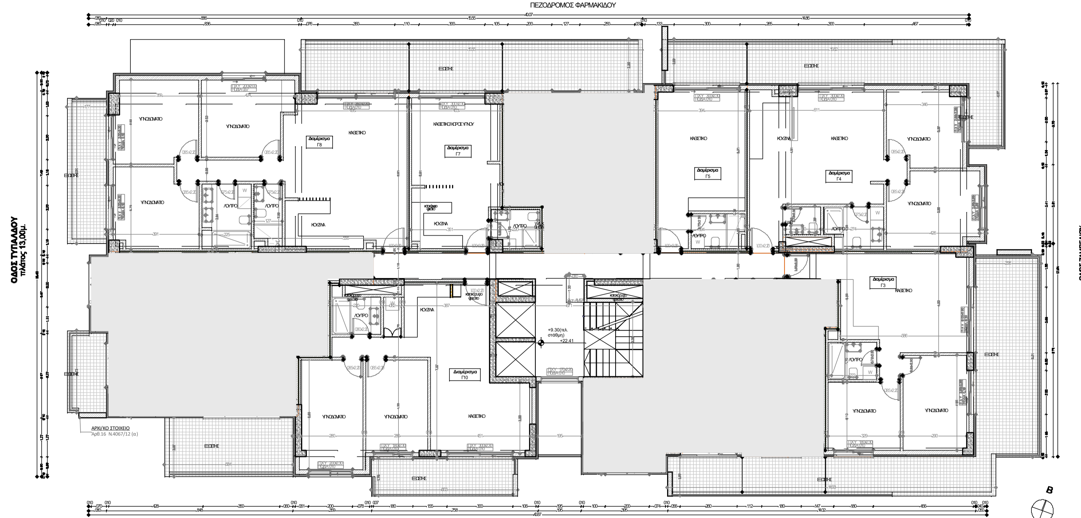
ΚΑΤΟΨΗ 3ου ΟΡΟΦΟΥ ΚΛΙΜΑΚΑ 1:100
