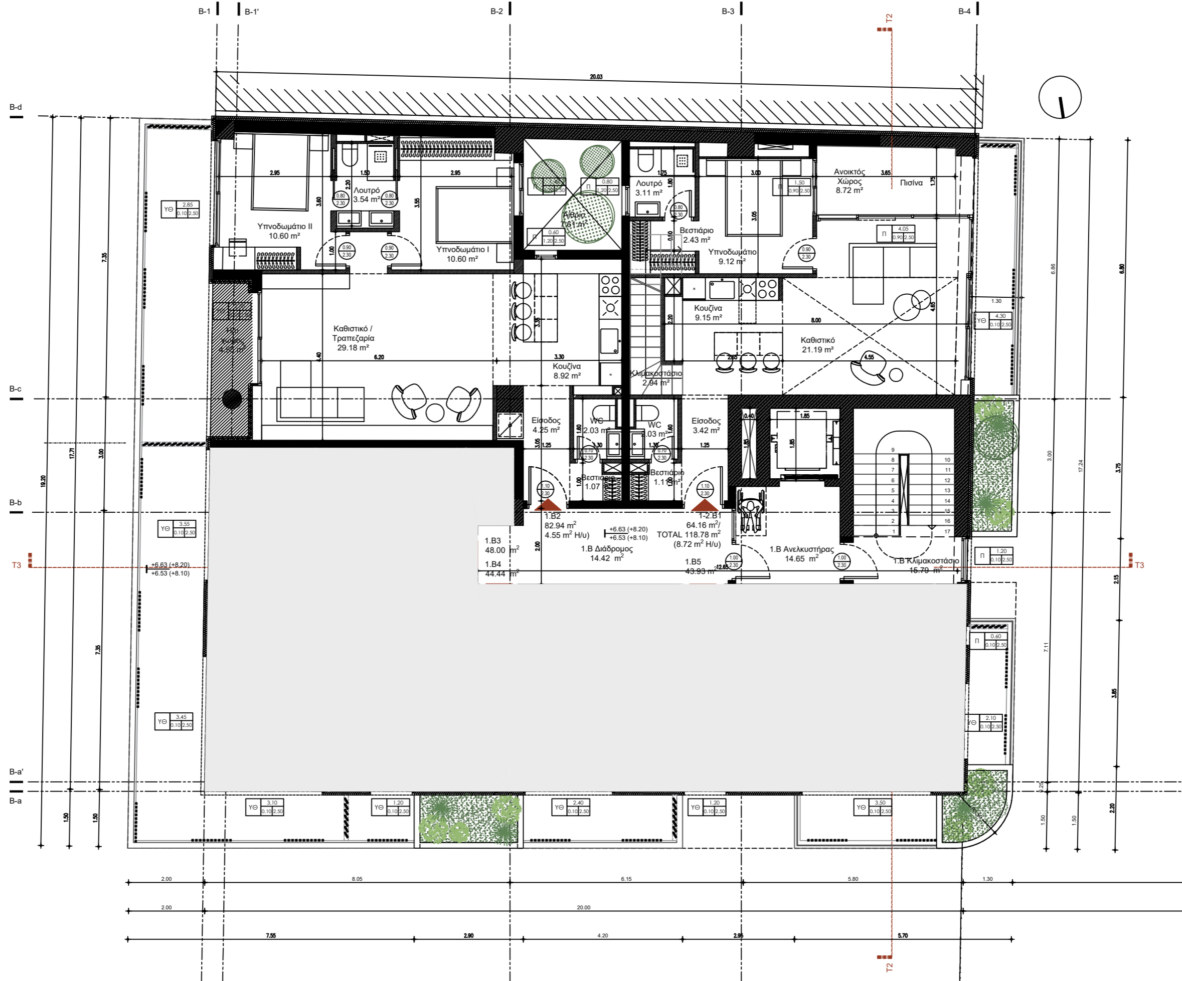
ΚΤΙΡΙΟ Β ΚΑΤΟΨΗ 2ου ΟΡΟΦΟΥ ΚΛΙΜΑΚΑ 1:100
