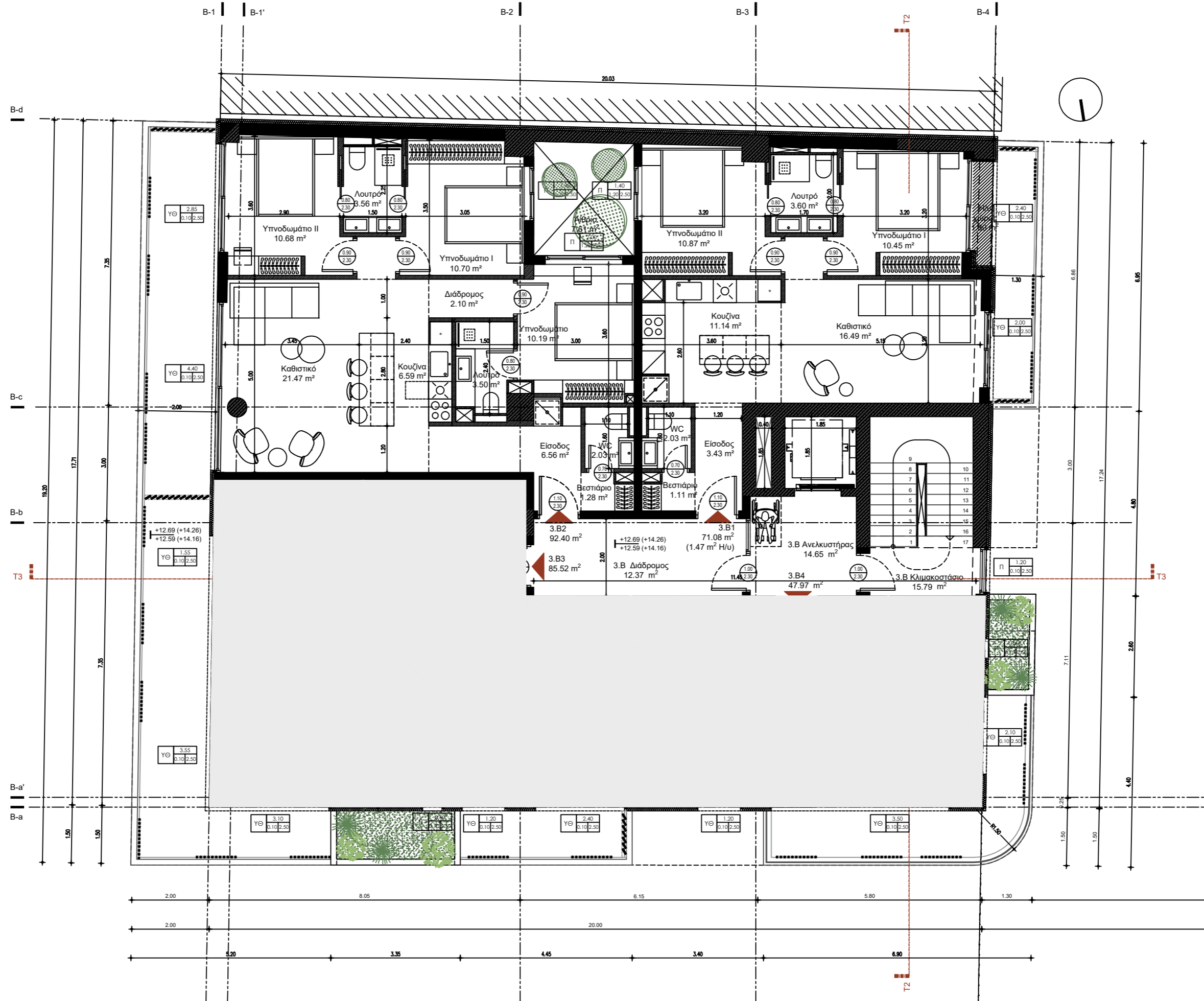
ΚΤΙΡΙΟ Β ΚΑΤΟΨΗ 4ου ΟΡΟΦΟΥ ΚΛΙΜΑΚΑ 1:100
