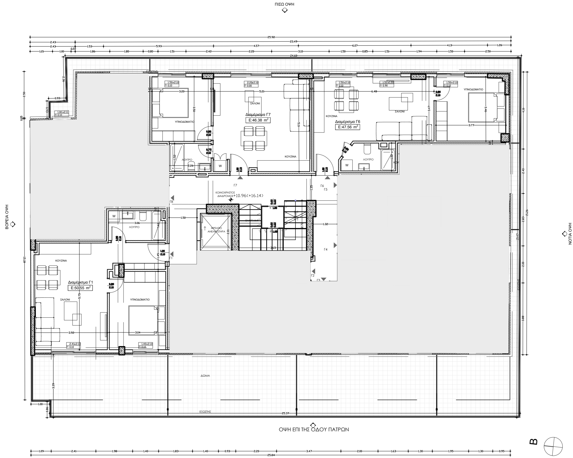
ΚΑΤΟΨΗ 3ου ΟΡΟΦΟΥ (Α' ΕΣΟΧΗ) ΚΛΙΜΑΚΑ 1:100
